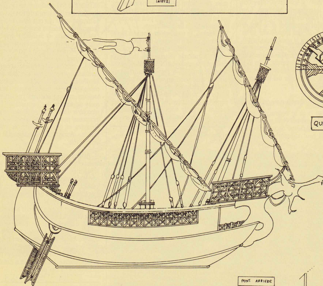
NEF MARCHANDE
